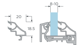
con junquillo 17-20mm S60 Acristalamiento 8-10mm
