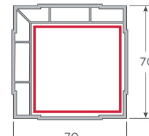
Esquinero 90° - 70mm Corredera
