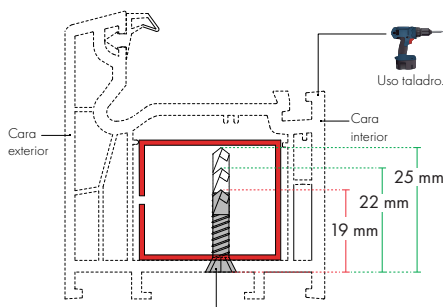
SECCIÓN TRANSVERSAL - EN USO CON MEDIDAS
