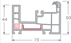
Marco Monorriel Corredera Andes con apoyo cerradero 7x7 - M
