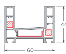
Marco Doble Riel Corredera Andes con Apoyo cerradero 7x7 - M
