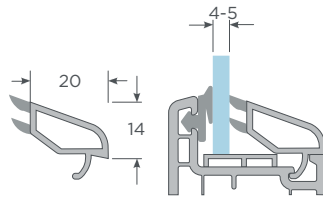
Junquillo monolítico 4-5mm Andes
