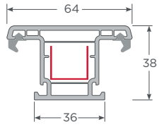
Poste T & Hoja exterior Andes S38
