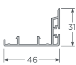
Traslapo Andes 54 Blanco
