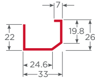
Ref. múltiple inclinación 2mm RFMLT20
