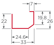
Ref. múltiple inclinación 1.2mm RFMLT12
