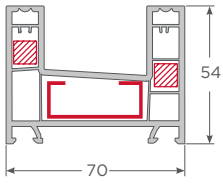
con Apoyo cerradero 9x9 Marco doblerial
