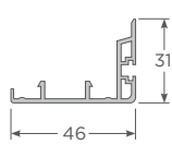
Traslapo ventana corredera
