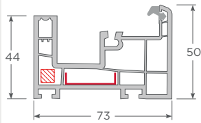
con Apoyo cerradero 7x7 Marco corredera monoriel
