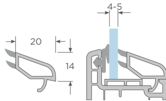
Junquillo monolítico 4-5mm
