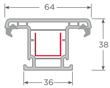
Poste T & Hoja exterior
