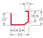
Ref. New Múltiple 2mm - TC PL-CMP-TC-MLT-2
