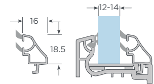
Con junquillo 22-24 S60 Acristalamiento 12-14mm
