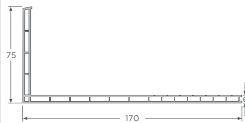
Ángulo Revestimiento 75/170mm
