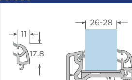
Con junquillo 17-20 Sliding Acristalamiento 26-28
