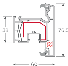
con Apoyo cerradero 9x9 - M Hoja Ventana Exterior
