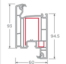
con Ref. bisagra hoja puerta S60 1.2 mm
