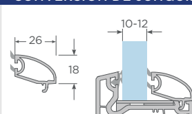
Con junquillo 4-5 Sliding Acristalamiento 10-12
