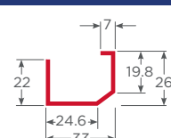
Ref. New Múltiple 2mm - TC PL-CMP-TC-MLT-2
