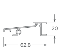
Zapata Puerta Aluminio 60mm - 3mt
