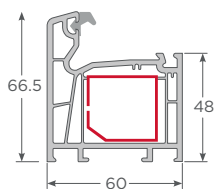
Marco Fijo S60
