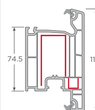
Hoja Puerta Exterior
