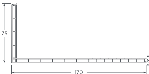
Ángulo de Revestimiento 75/100mm
