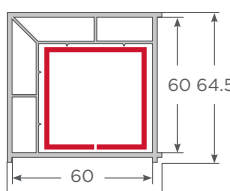
Esquinero 90° 60mm S60
