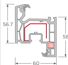
con Apoyo cerradero 7x7 - M Hoja Ventana Interior
