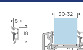
Con junquillo 20-22 Sliding Acristalamiento 30-32
