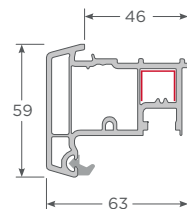
Poste Inversor o Batiente
