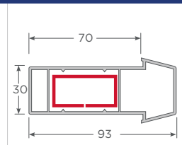
Inercia T
