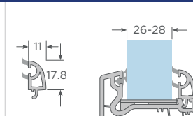
Con junquillo 17-20 Sliding Acristalamiento 26-28
