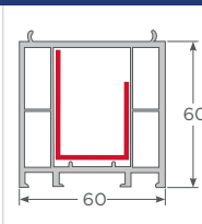
Utiliza Ref. Hoja Puerta corredera 98 Perfil Elevación S60
