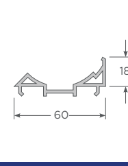
Adaptador Rótula S60
