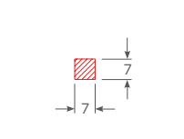
Apoyo Cerradero 7x7 - M HL-ACC-7X7-APOC-MA
