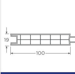
Placa Machiembre 19
