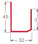
Ref. Hoja Puerta Corredera c/inclinación 2mm - TC PL-S60-TC-H98-2
