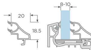
Con junquillo 17-20 S60 Acristalamiento 8-10mm
