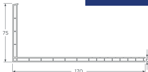
Ángulo Revestimiento 75/170mm
