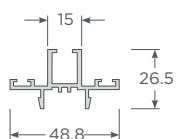
Adaptador Cuarta Hoja con Felpa
