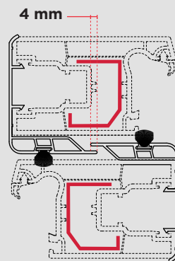
TRASLAPO HOJA - 80
