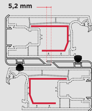
TRASLAPO HOJA - 98
