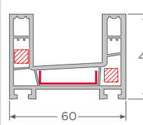
Marco Doble Riel Corredera Andes
