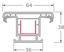
Poste T & Hoja exterior Andes S38
