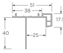
Aleta Siding Marco Fijo Andes
