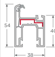
Hoja Andes 54 Blanco
