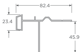
Traslapo Andes 54 Blanco
