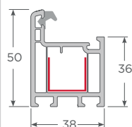
Marco Fijo Andes S38
